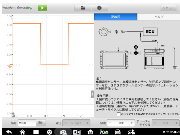
図 7-8 配線図とヘルプ画面のサンプル
