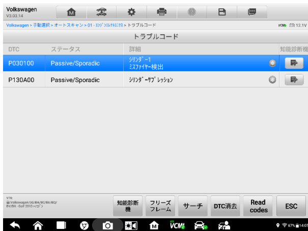
図 5-14 「故障コード」画面のサンプル
