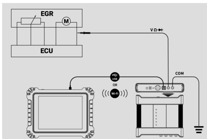
図 7-12 アクチュエータドライブの接続図のサンプル
