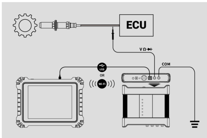
図 7-13 方形波接続図のサンプル
