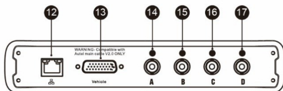
図 2-6 Maxi Flash VCM1 底面図
