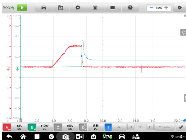
図 7-10 基準信号の波形表示のサンプル
