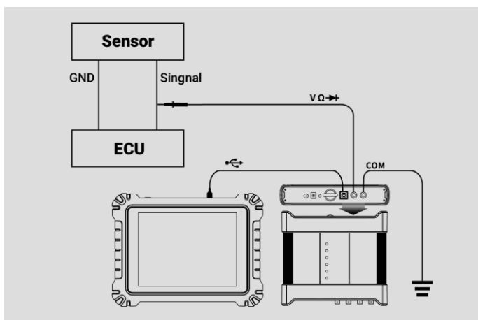
図 7-16 任意波形接続図のサンプル
