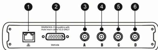
VCM1 底面図
