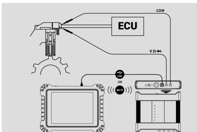
図 7-14 方形波 (X + Y) 接続図のサンプル
