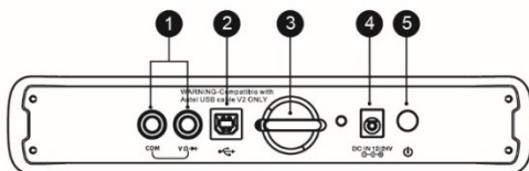
VCM1 上面図
