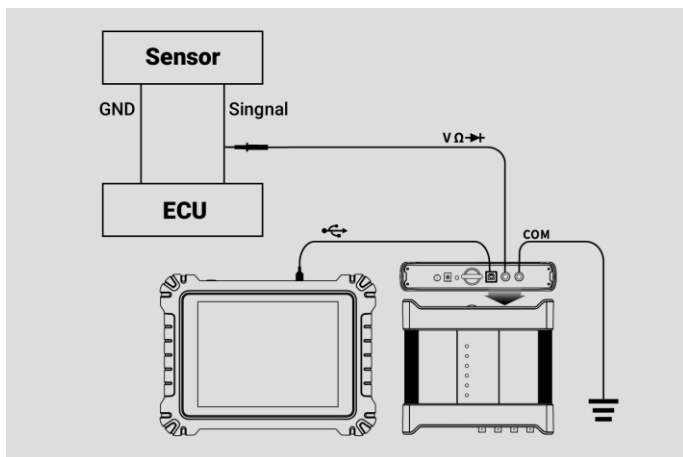
図 7-15 三角波の接続図のサンプル
