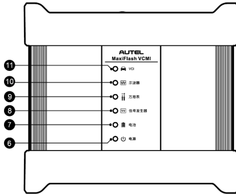
VCM1 正面図
