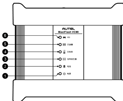
VCMI 正面図
