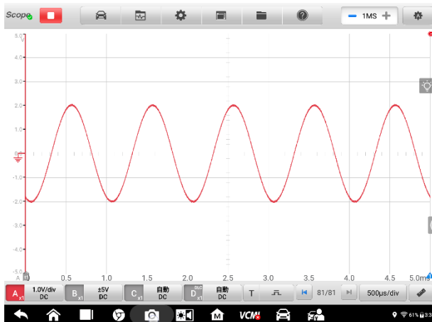
図 7-50 振幅設定図のサンプル (DC 5V)
