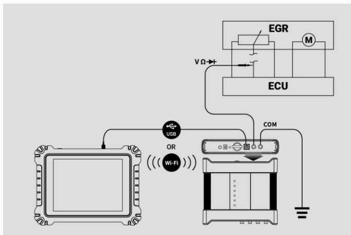
図 7-11 DC 電圧接続図のサンプル
