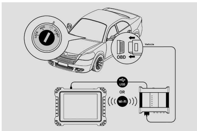
図 7-60 DLC 接続図のサンプル
