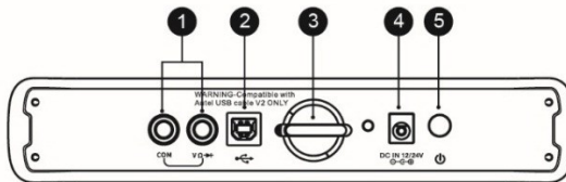
図 2-4 Maxi Flash VCMII 上面図
